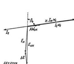
Fig. 6. Stromwandlerdiagramm für Ueberstrom.
