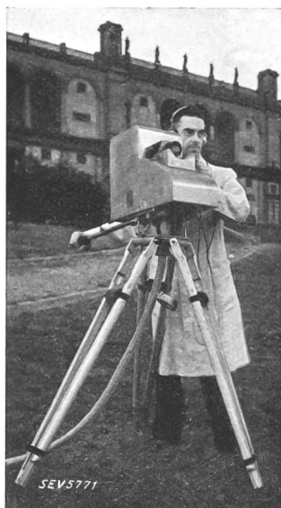
Fig. 5. Emitron-Kamera.
