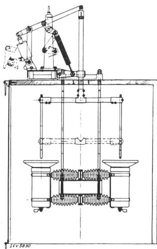
Fig. 11. Topfschalter Oerlikon (1904—1908.)
