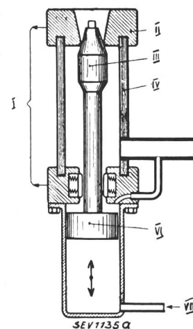
Fig. 15. Prinzip der modernen Druckgasschalter.
