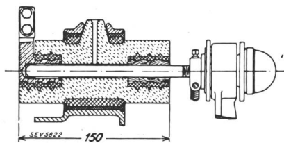
Fig. 1. Schalttröhre des Röh- renschalters Westing- house (1896). (Aus Vogelsang: Geschichtliche Einzel- darstellungen aus der Elektrotechnik, Berlin 1929.)
