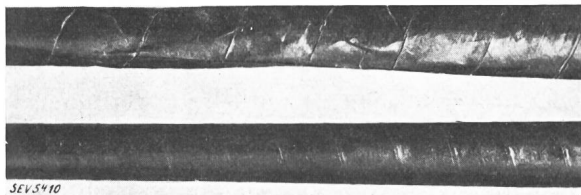
Fig. 4 (oben). Fig. 5 (unten). Sektorkabel alter (oben) und neuer (unten) Fabrikation.
