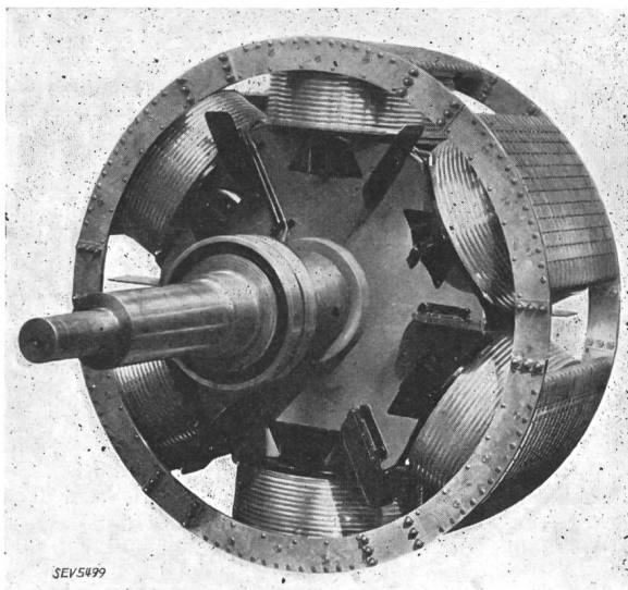
Fig. 1. Roue polaire équipée avec un amortisseur.
