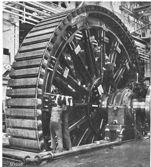
Fig. 3. Rotor d'alternateur triphasé en cours de montage.
