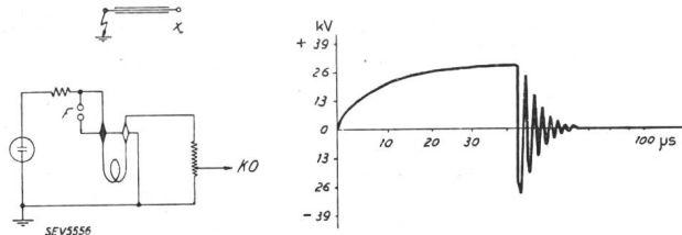
Fig. 3. Oscillation propre de 100 m de câble.
