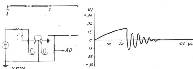
Fig. 5. Oscillation de 200 m de câble relié à 900 m de ligne aérienne.
