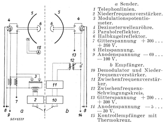
Fig. 21. Schema einer Dezimeterwellenverbindung.
