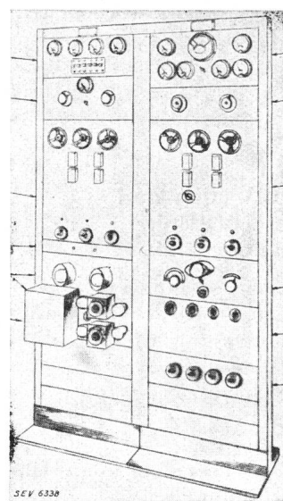
Fig. 22. Dezimeterwellenanlage im Stationsgebäude in Lympne. 1 Verstärker-Messinstrumente. 2 Modulationsregulierung. 3 Regulierung des Dezimeterwellensenders. 4 Kontrollanschlüsse. 5 Niederfrequenzverstärker (Sender). 6 Niederfrequenzverstärker (Empfänger). 7 Messinstrumente zur Ueberwachung der Dezimeterwelle. 8 Demodulator. 9 Regulierung des Dezimeterwellenempfängers. 10 500-kHz-Oszillator. 11 Verstärker-Netzanschluss. 12 Netzschalter.
