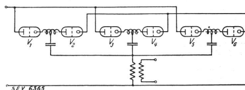
Fig. 5. Speicherwechselrichter für hohe Frequenzen.
