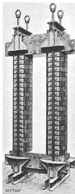
Fig. 1. Eisenkörper einer 5650-kVA-Oerlikon-Erdschlusspule.
