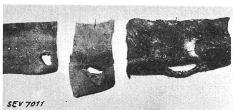
Fig. 6. Enveloppes de câbles placées dans des zorès et détériorées par des coups extérieurs.
