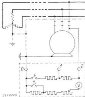
Fig. 4. Schema zum normalen Erdungsprüfer.
