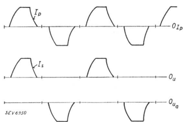
Fig. 1. Schematische Darstellung des zeitlichen Verlaufs der Stromkurven in Primär- und Sekundärwicklungen. O_{tp} Nulllinie d. Kurve des Primärstromes. O_u Nulllinie, Phase u . O_{ua} Nulllinie, Gegenphase u_a .
