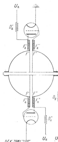
Fig. 5. Schema des Einbaus zweier Röhren in einen Kugelkreis.
