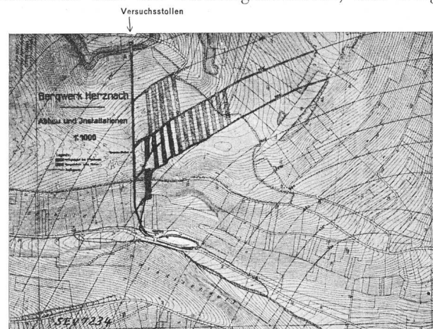
Fig. 17. Bergwerk Herznach: Abbau- und Installations-Plan. ■ Abgebaut bis 1. Februar 1938. ▨ Zum Abbau vorgesehen. / Isohypsen. Aequidistanz 5 m. Der Abbau erfolgt zwischen den Isohypsen 460—465—470 m ü. M.
