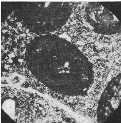
Fig. 8. Oolith mit konzentrisch-schaliger Struktur. Oolith mit Quarzkern.
