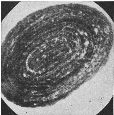
Fig. 8. Oolith mit konzentrisch-schaliger Struktur. Oolith mit Quarzkern.
