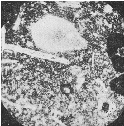
Fig. 7. Schwarz: Oolithe. Weiss: Grundmasse aus Quarz und Kalkspat. Grundmasse mit Fossilbruchstücken.
