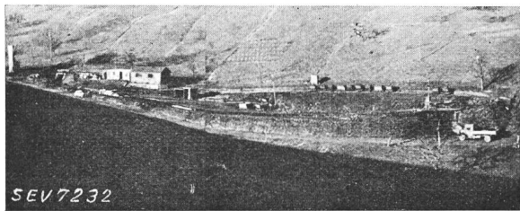
Fig. 18. Bergwerk Herznach. Installationen über Tag und Verladerampe.
