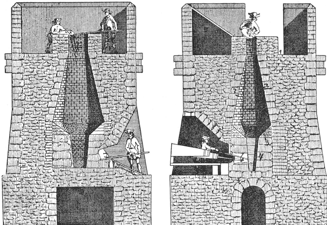
Fig. 20. Holzkohle-Hochofen.
