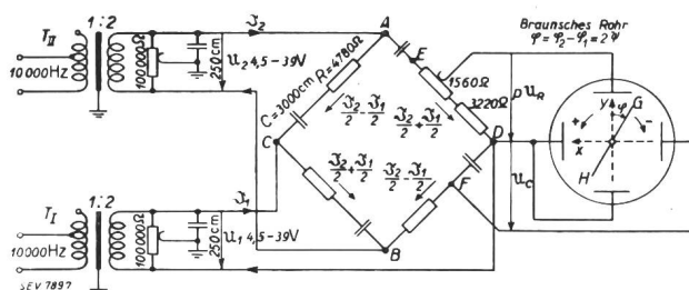
Fig. 1. Schaltbild der Messanordnung.
