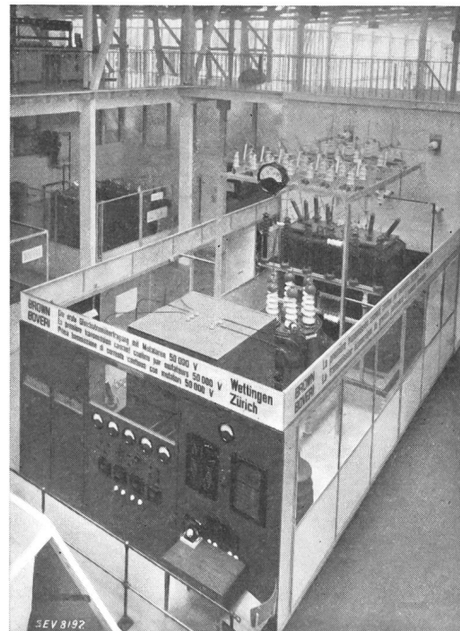
Fig. 2. Gleichstrom-Uebertragung Wettingen-Zürich.
