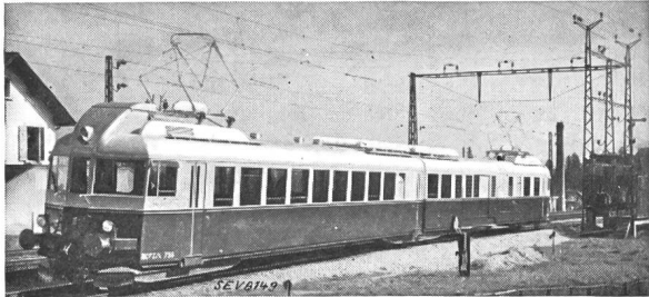
Fig. 1. Leichttriebzug Typ BCFZe 4/6 der BLS. Zugkraft einständig 3320 kg bei 68,5 km/h. Höchstgeschwindigkeit 110 km/h.
