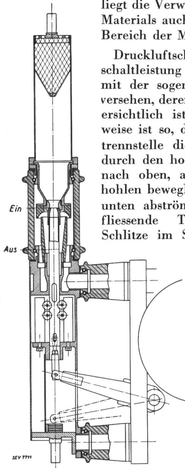
Fig. 14. Druckluftschalter mit keramischer Isolation für feuchte Räume. Der Schalter besitzt Doppeldüse.
