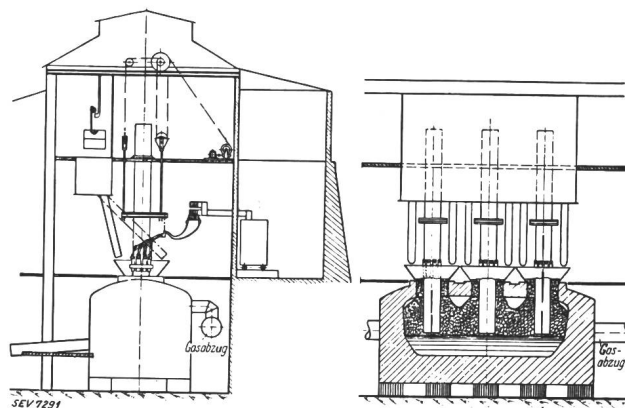
Fig. 2. Tysland-Hole-Ofen.
