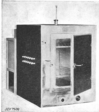
Fig. 15. Konditionierschrank (Vorderseite).
