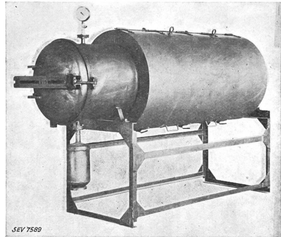
Fig. 16. Vakuumkessel.
