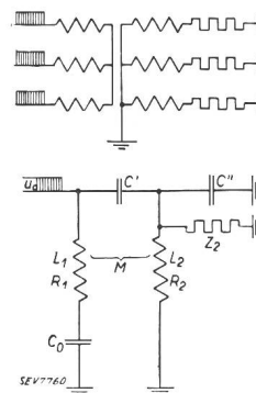
Wicklungs- und Ersatzschema für die dreiphasig angestossene Sternwicklung.
