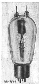
Fig. 3 (oben). Ultrakurzwellen- Senderöhre TB 1/60.
