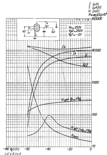
Fig. 6. Röhre EF 50.
