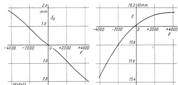
Fig. 3. Verschiebung der «Nulllinie» in Funktion der Gleichspannung beider parallelgeschalteter Ablenkplatten.
