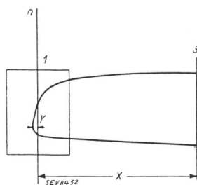
Fig. 2. Auswertung der Oszillogramme bei der Kompensations- schaltung. X Ablenkung infolge der Gleich- strom-Schubspannung X' . Y Restablenkung entsprechend Restspannung Y' . X' + Y' Gesuchte Stoßspannung U . n Nulllinie mit geerdeten Ab- lenkplatten des KO. s Stosslinie. 1 Schirm.
