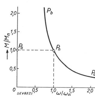
Fig. 3. Idealer Gleichstrom-Reihenschlussmotor.
