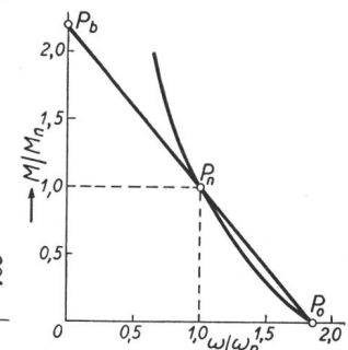
Fig. 4. Allgemeine Idealturbine.
