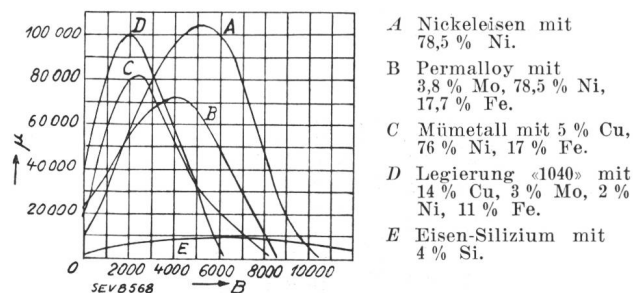
Permeabilitätskurven für magnetische Werkstoffe mit hoher Permeabilität.
