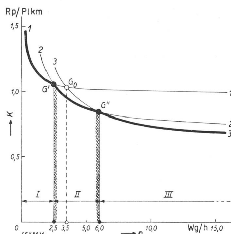
Fig. 1. Abgrenzung der Anwendungsgebiete. 1 Autobus. I Gebiet des Autobus. 2 Trolleybus. II Gebiet des Trolleybus. 3 Tramway. III Gebiet des Tramway.
