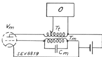
Fig. 4. Modulatorschaltung. V_m Modulationsröhre, O Oszillator.
