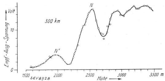
Fig. 9. Gemessene Vertikaldiagramme. (Sender N, \lambda = 4,1 m) 12. 7. 1935.
