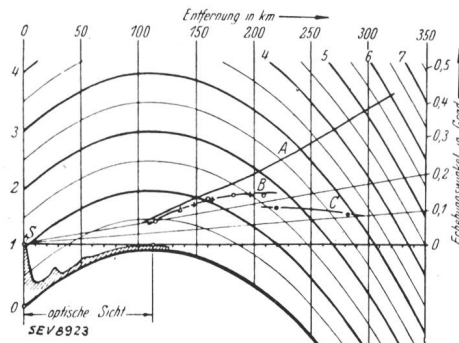
Fig. 4. Profilschnittdarstellung zum Vergleich des gerechneten und gemessenen Strahlen- verlaufs. Sender B, \lambda = 7,17 m. S Sender, A gerechneter Verlauf, B, C ge- messener Verlauf des untersten Maximums des Vertikaldiagramms. Die Rechnung gilt für geradlinigen Strahlenverlauf. Messungen am 30. 9., 3. 8., 11. 10. 1935.
