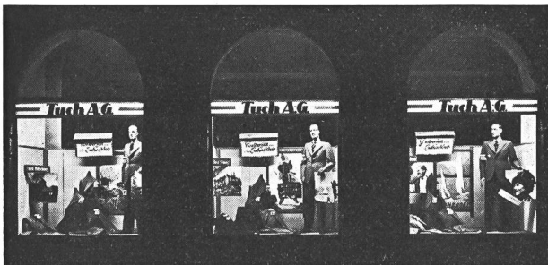
Fig. 11. Tuch A.-G., Luzern. Schaufensterbeleuchtung mittelst Hochspannungsleuchtstoff- röhren, 65 Watt, 2000 lm. Pro Schaufenster je zwei Röhren, eine mit tageslichtweisser, eine mit rötlichweisser Lichtfarbe.
