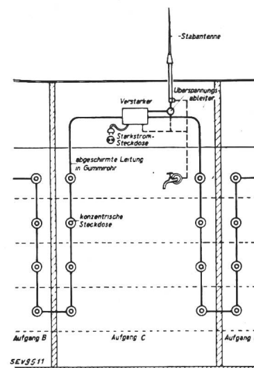
Fig. 7. Schaltschema einer Gemeinschafts- antennenanlage mit Verstärker für 5 Aufgänge mit je 8 Wohnungen.
