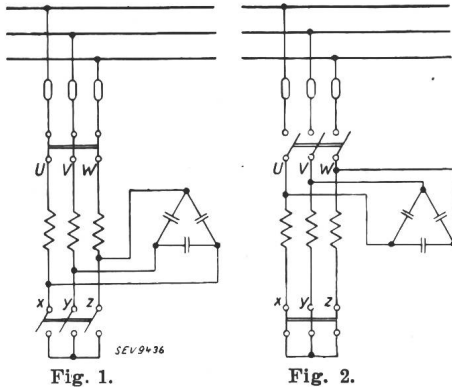
Fig. 1. Fig. 2. Moments dangereux pendant le démarrage de moteurs à couplage étoile-triangle compensés individuellement.
