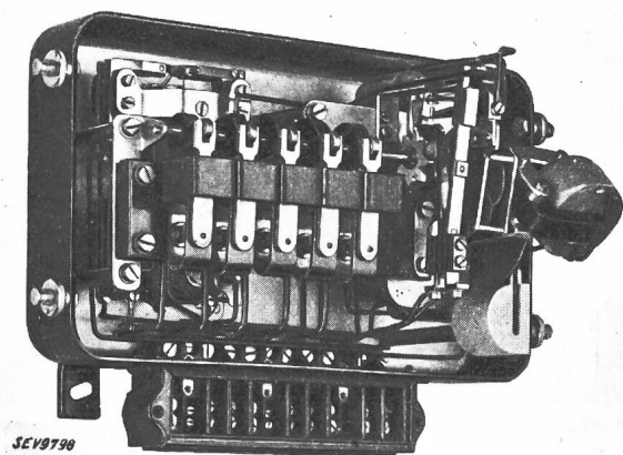
Fig. 2. Blindlast-Regelanlage: Stufenschalter.
