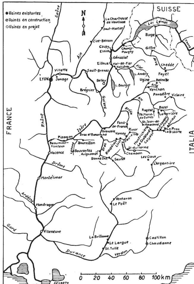
Fig. 3. Carte synoptique du bassin du Rhône avec l'indication des principales usines hydroélectriques françaises.
