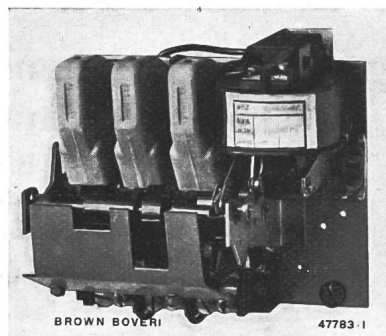
Fig. 1. Magnetbetätigter Kleinschalter ohne Gehäuse.
