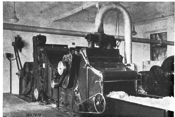
Fig. 11. Baumwoll-Voröffner-Gruppe.
