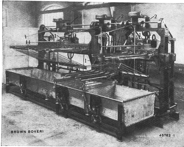
Fig. 5. Stranggarn-Färbemaschine. Trogseite.
