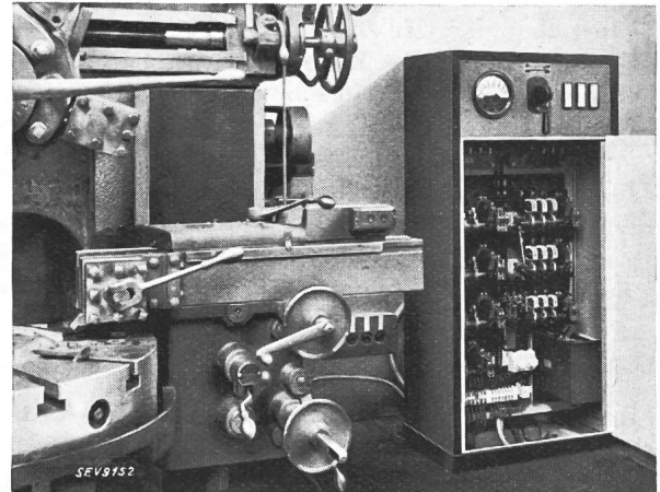
Fig. 3. Karusselldrehwerk mit Antrieb durch polumschaltbaren Motor und Schützensteuerung.
