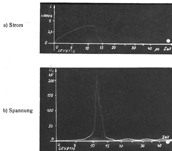
Fig. 9. Kathodenstrahl-oszillogramme eines Durchschmelzversuches eines Silberdrahtes in Quarzsand bei Stoss.
