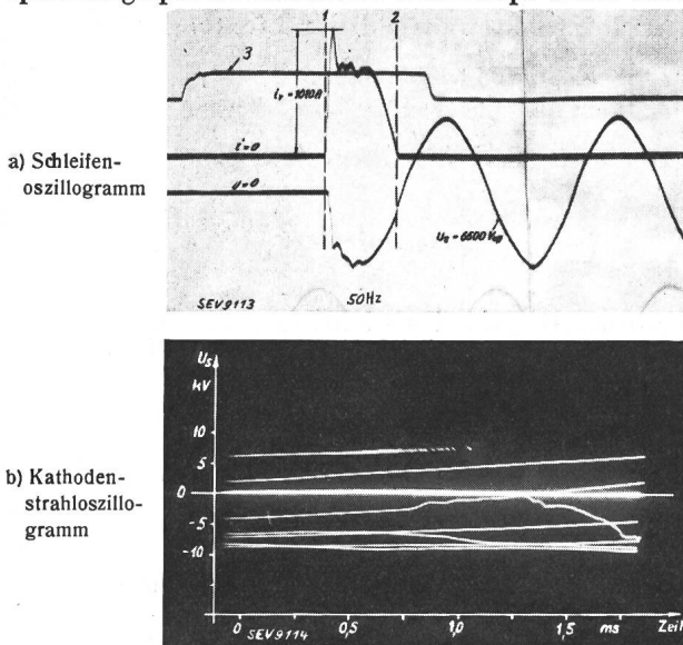
Fig. 8. Abschaltung durch progressiv schaltende Sicherung.
