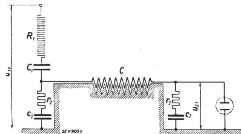
Fig. 5. Schéma du diviseur retardateur suivant M. Burch.
