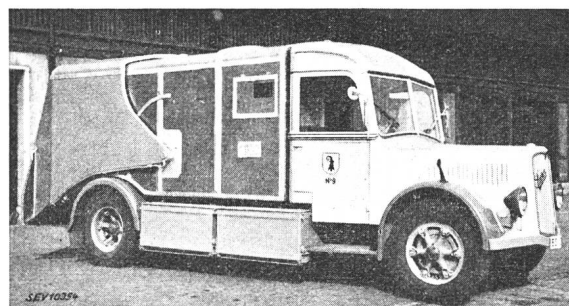
Fig. 2. Elektrofahrrad für die Kehrichtabfuhr max. Nutzlast 2820 kg
