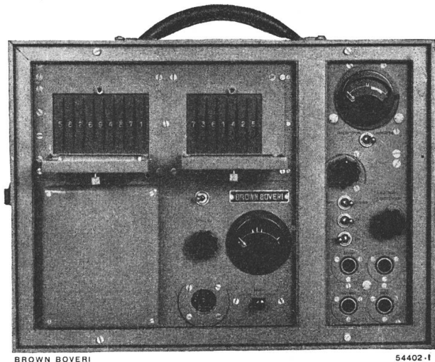
Fig. 2. Anwendung von Panzerholz in der Hochfrequenztechnik. Panzerholzgehäuse einer tragbaren Schlüsselungsapparat.
