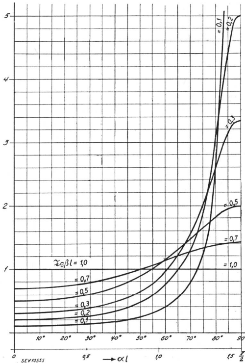
Fig. 1. Tangens hyperbolicus
