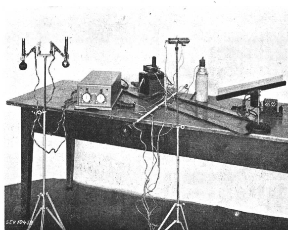
Fig. 2. Elektrische Messausrüstung.
