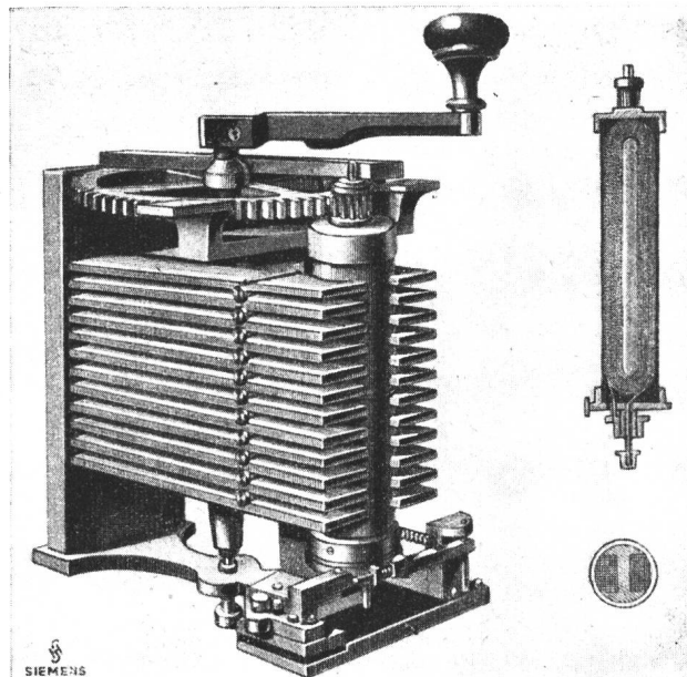
Fig. 1. Magnetoelektrischer Zeigertelegraph von Werner Siemens mit Doppel-T-Anker (1856).
