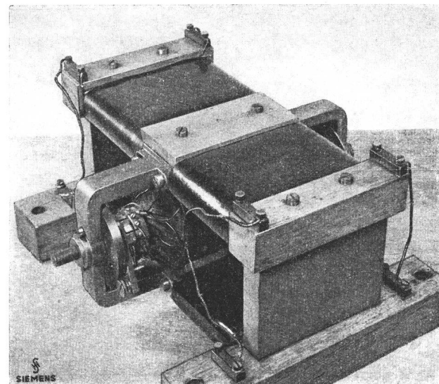
Fig. 5. Erste Trommelankermaschine, Original im Reichspostmuseum Berlin (1872).
