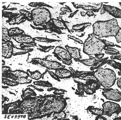
Fig. 3. Molybdän-Silber-Verbundmetall. Mikrostruktur, Vergr. 200fach.
