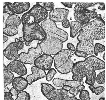
Fig. 5. Wolfram-Kupfer-Verbundmetall. Mikrostruktur, Vergr. 200fach.
