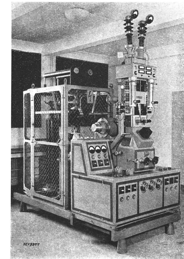
Fig. 7. Doppelkathodenstrahl-oszillograph.
