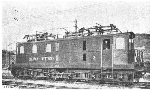
Fig. 4. Lokomotive Nr. 3.
