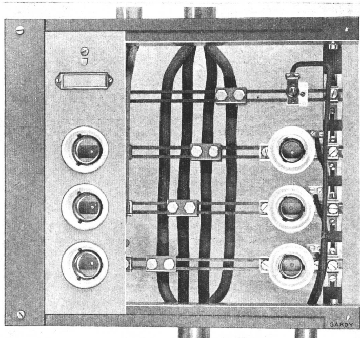
Links: Gardy U.P.-Apparate-Zusammenbausystem für Selbstkombination.
