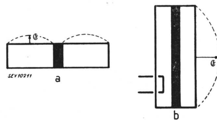
Fig. 3. Hohlraumresonatoren
