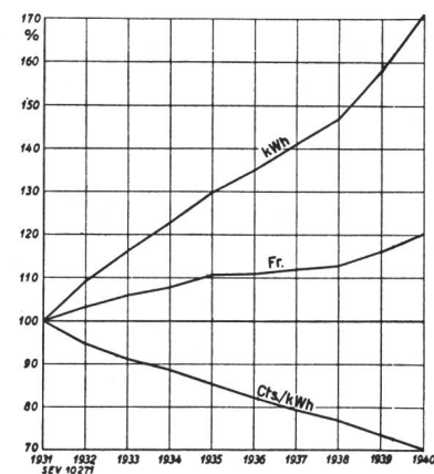
Fig. 11. Entwicklung 1931...1940 des Ver- brauches aller Haus- altanwendungen, der entsprechenden Einnahmen der Werke und der er- zielten mittleren Energiepreise.
