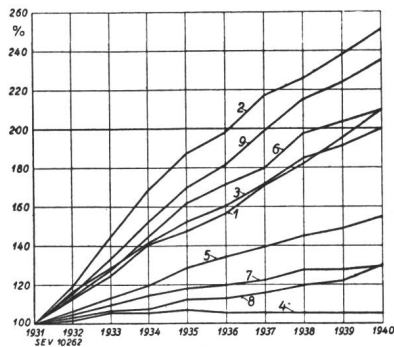
Fig. 1. Entwicklung der Zahl der Anschlüsse pro Einwohner 1931...1940 (1931 = 100).
