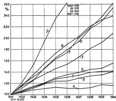
Fig. 2. Entwicklung der Anschlusswerte pro Einwohner 1931...1940 (1931 = 100).
