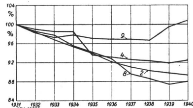
Fig. 3. Entwicklung des mittleren Anschluss- wertes pro Apparat 1931...1940 (1931 = 100).
