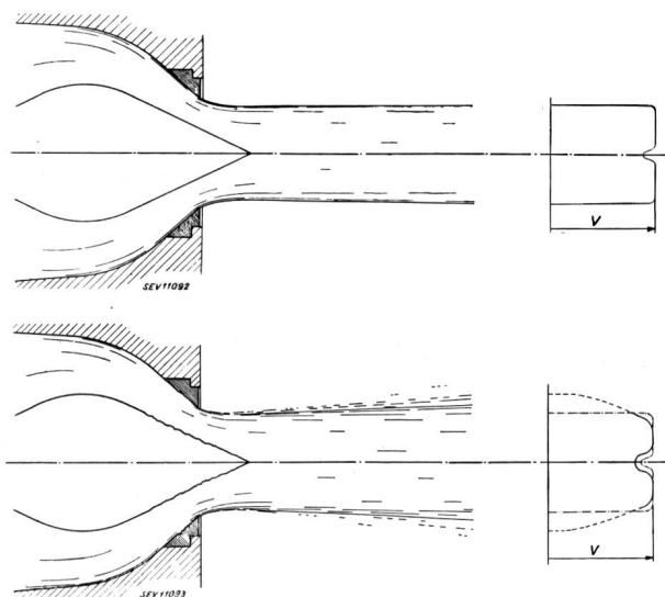
Fig. 2 (oben) und Fig. 3 (unten). Ausbildung des Wasserstrahles durch unabgenutzte (oben) und abgenutzte (unten) Nadel und Düse v Strahlgeschwindigkeit.
